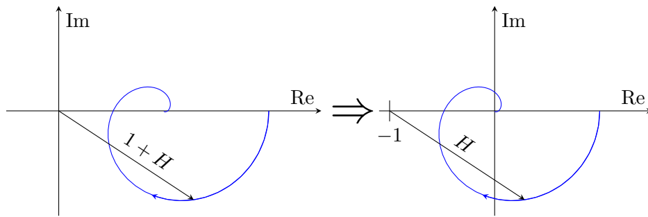
Abbildung 4: Ortskurve 1 + H(i\omega) eines asymptotisch stabilen geschlossenen Kreises (links) und H(i\omega) des entsprechenden asymptotisch stabilen offenen Kreises (rechts).
