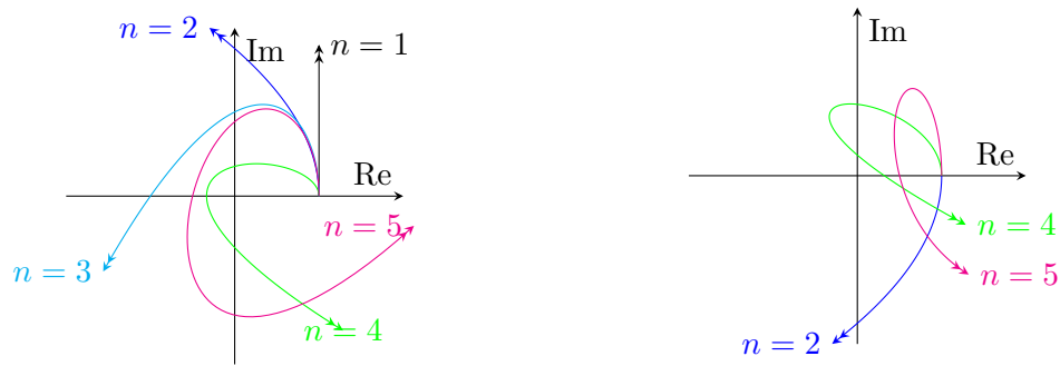
Abbildung 2: CLM-Ortskurven asymptotisch stabiler (linkes Bild) und instabiler (rechtes Bild) Systeme
