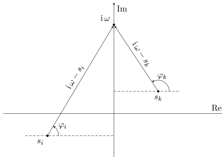
Abbildung 1: Phasenwinkel für eine Nullstelle s_i in der linken und eine Nullstelle s_k in der rechten Halbene der komplexen Zahlenebene.
