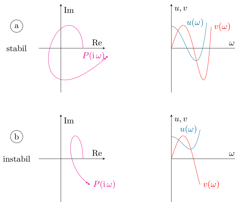
Abbildung 3: Verlauf der CLM-Ortskurve P(i\omega) sowie u(\omega) und v(\omega) für (a) ein asymptotisch stabiles und (b) ein instabiles System.
